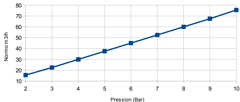
Consommation d'Air (Air à 0° C)
